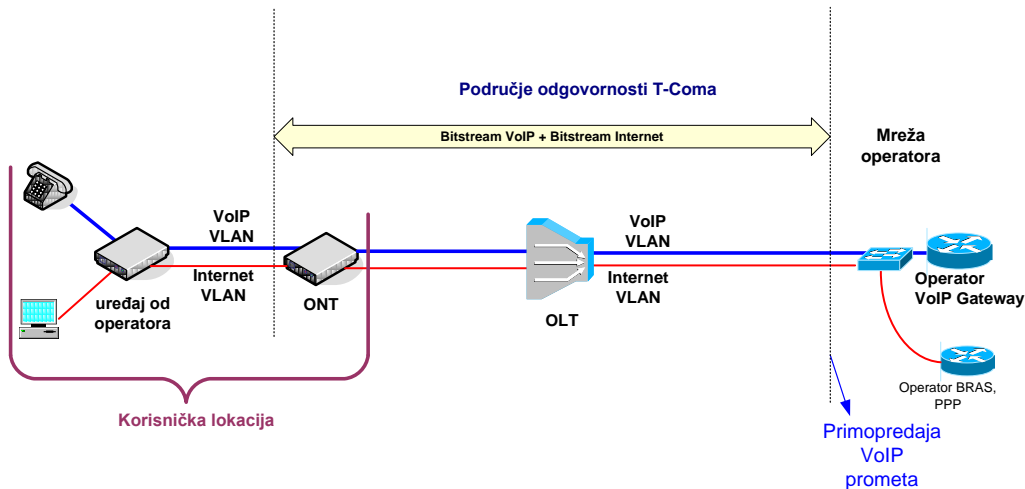
Slika 18. Veleprodajni širokopojsni pristup za pružanje VoIP usluge preko FTTH pristupa (GPON) na OLT razini
