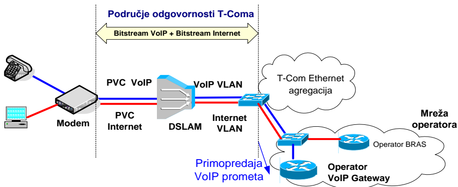
Slika 19. Veleprodajni širokopojsni pristup za pružanje VoIP usluge preko ADSL/VDSL pristupa na DSLAM razini
